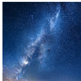
droga mleczna
