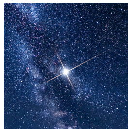
gwiazda
