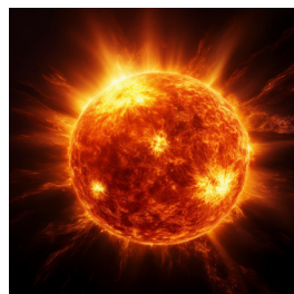
Słońce
