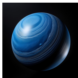
Neptun
